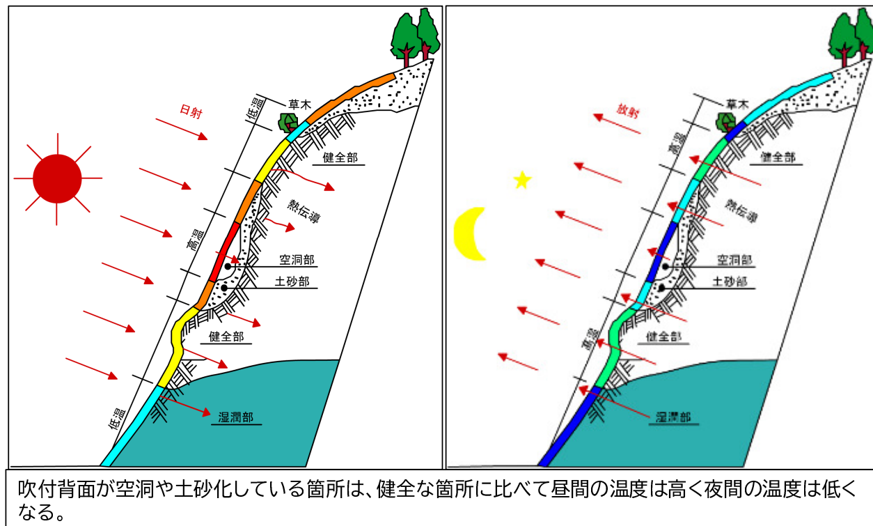
図1: 熱赤外線調査概念図
